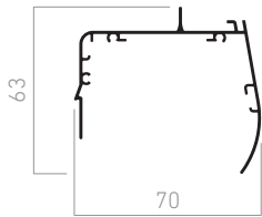
Semicajón 90
