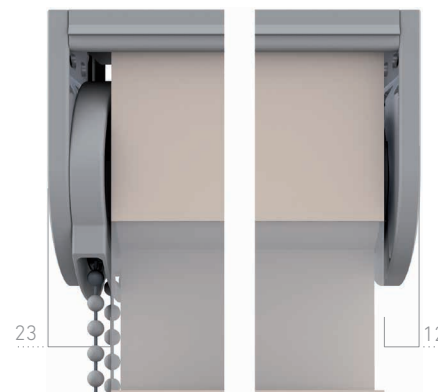
Sistema básico barra estabilizadora
