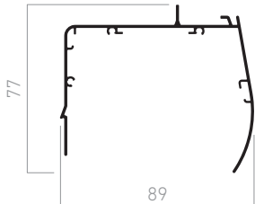
Barra estabilizadora
