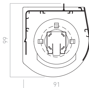
Sistema semicajón 90
