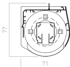
Sistema semicajón 70
