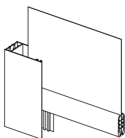
Terminal interior guía Inter bottom weight Lame finale intérieur et coulisse
