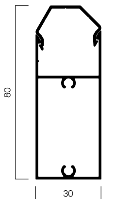
Sezione Lama R-80 Fissa
