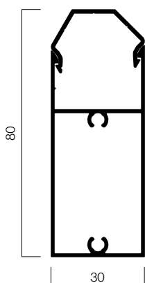
Sección Lama R-80 Fija
